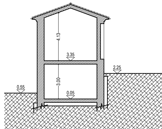
SEZIONE A-A
