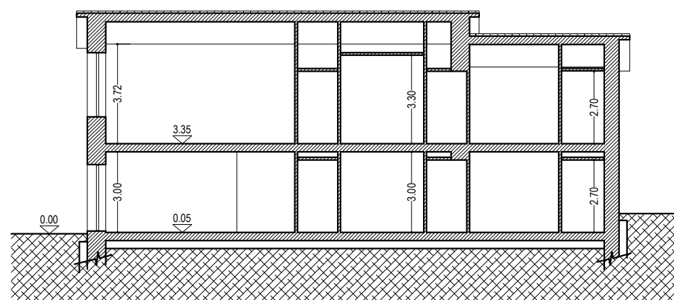
SEZIONE B-B
